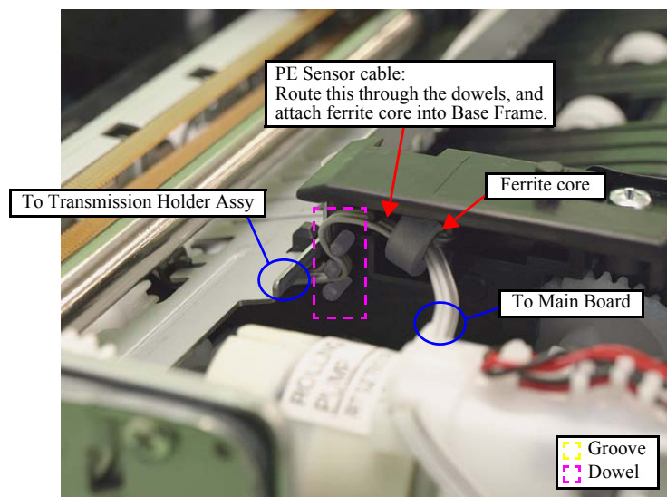
Figure 4-256. PE Sensor Cable
